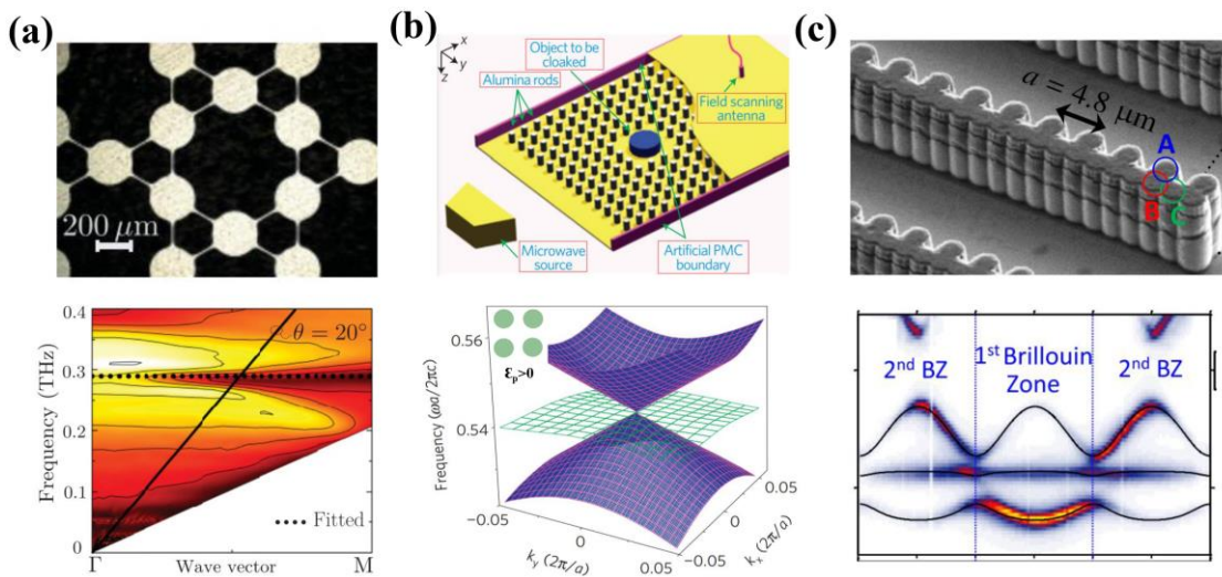
图 2 光子系统中平带研究的典型实例 (a) 上图为表面等离子激元平带的金属 Kagome 超构材料，下图为对应的太赫兹波透射图，存在一个全角度的无辐射平带（水平虚线所示） [48] ；(b) 四方结构的全介质零折射率超构材料实现隐身效应实验装置，下图为适当介质参数时得到的四方结构色散关系，含有一个狄拉克锥与一个无色散平带 [50] ；(c) 一维“枕”型结构的微柱光学腔及其色散关系，中间为平带 [51]
