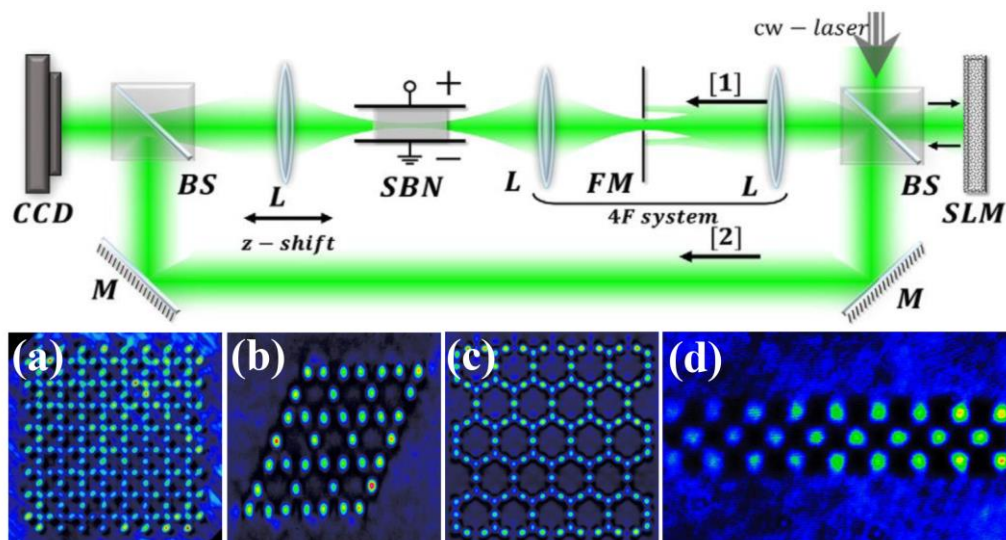
图 5 连续激光直写技术制备不同平带光子晶格. 第一排为实验光路图: SLM, 空间光调制器; BS, 分光棱镜; FM, 傅里叶掩模板. 第二排为典型的直写光子晶格: (a) “胡须”边界 (“bearded” edges) 的 Lieb 光子晶格 [89] ; (b) 平滑边界的 Kagome 光子晶格 [90] ; (d) 超级蜂窝晶格 [91] ; (e) 横向折射率梯度变化的菱形光子晶格 [92] .
