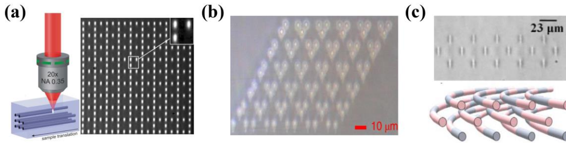
图 3 利用飞秒激光直写技术制备的平带光子晶格 (a) 用于研究平带局域模式的 Lieb 光子晶格 [64,65] ; (b) 用于研究拓扑角态的 Kagome 光子晶格 [66] ; (c) 用于实现 Aharonov-Bohm 效应的纵向弯曲菱形光子晶格 [67,68]
