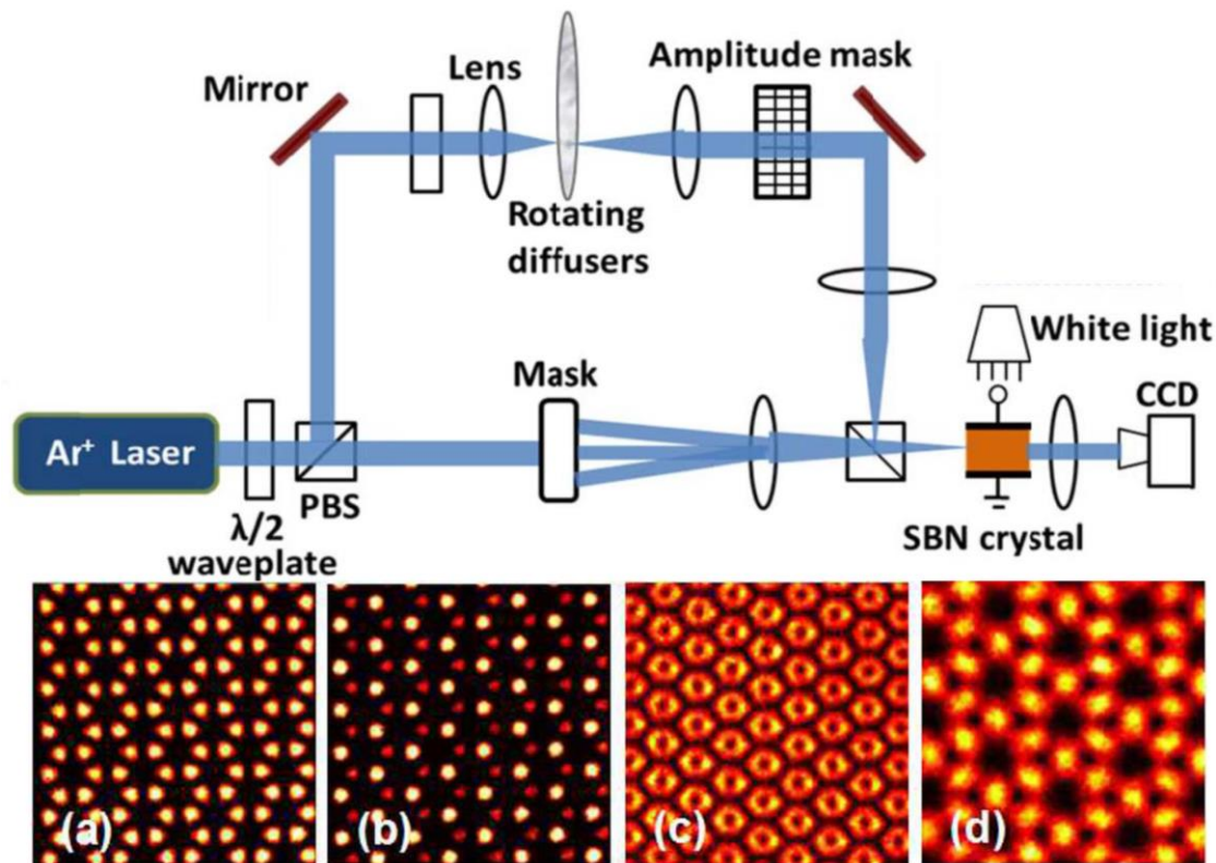
图 4 多光束干涉光诱导技术制备光子晶格 [80,83] . 第一排: 实验光路图. PBS, 偏振分光棱镜; Mask, 掩膜板; SBN, 铌酸锶钡晶体. 第二排: 实验制作的典型光子晶格 (a) 蜂窝型光子晶格; (b) 对称破损的蜂窝型光子晶格; (c) 涡旋晶格; (d) Kagome晶格
