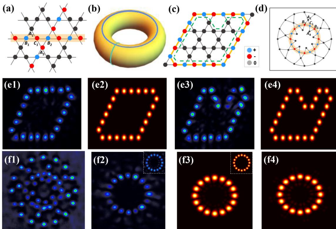
图 8 (a) Kagome 晶格中两种不可压缩环形态示意图；(b) 模拟无限 Kagome 晶格两个不可压缩环形态的圆环面；(c) 在平滑边界的 Kagome 晶格中两种稳定的平带边界局域模，橘黄色线代表模式一，绿色虚线代表模式二；(d) Corbino-Kagome 结构示意图，橘黄色圆环代表不可压缩的局域环形态。(e) 从左至右 (e1), (e2) 边界模式一的反相位输出与对应数值模拟结果；(e3), (e4) 边界模式二的反相位输出与对应数值模拟结果；(f1) 实验制备的 Corbino-Kagome 光子晶格；(f2), (f3)反相位激发的不可压缩环形态及其对应数值模拟结果；(f4) 40mm 传输时数值模拟结果. 图中所有插图均代表输入探测光. 同相位激发破坏所有平带局域模式的形成 [90]
