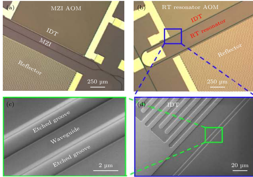
图 11 (a) M-Z 干涉仪型和 (b) 谐振腔型声光调制器的显微镜照片; (c) 光波导的 SEM 图像; (d) IDT 区域的 SEM 图像 [68]
