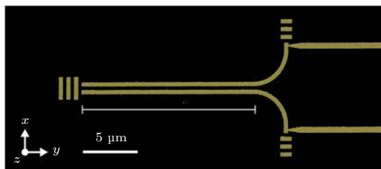
图 7 LNOI 片上等离子体电光定向耦合器的 SEM 图像 [51]
