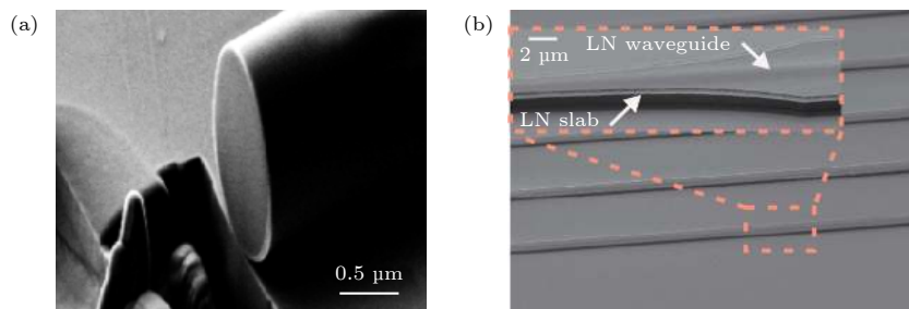
图 12 (a) 锥形单模光纤的 SEM 图像 [69] ; (b) 双层锥形模式转换器的 SEM 图像 [2]
