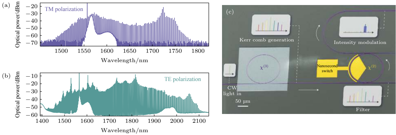
图 10 (a), (b) 宽带频率梳的产生, 即当抽运功率为 300 mW 且输入信号与 (a) TM 模和 (b) TE 模共振时, 产生的频率梳频谱; (c) LN 片上纳米光子学回路的 SEM 图像 [65]
