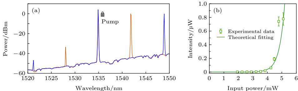
图 8 (a) 级联过程光谱, 其中抽运波长固定在 1534.9 nm, 信号光波长分别位于 1541.8 和 1548.9 nm; (b) LN 微盘中有有效的 FWM 过程, FW 闲频光功率依赖性和理论拟合, 信号光功率保持在 5 mW [55]
