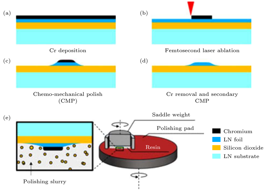
图 5 CMP 技术制备 LNOI 片上光子学器件流程图 (a) 磁控溅射沉积 Cr 薄膜; (b) 飞秒激光微加工制备待加工图案; (c) CMP 过程去除多余的 LN; (d) 使用 Cr 腐蚀剂去除蚀蚀掩模以及二次 CMP 过程; (e) CMP 仪器示意图 [38]
